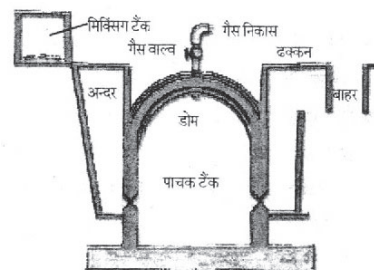
चित्र- गोबर गैस प्लांट
