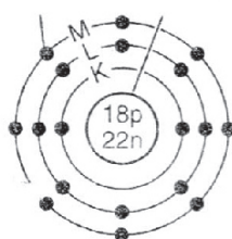
ऑर्गन-40
