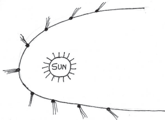
सूर्य के चारों ओर धूमकेतु की स्थिति
