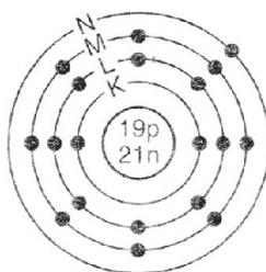
पोटैशियम-40
