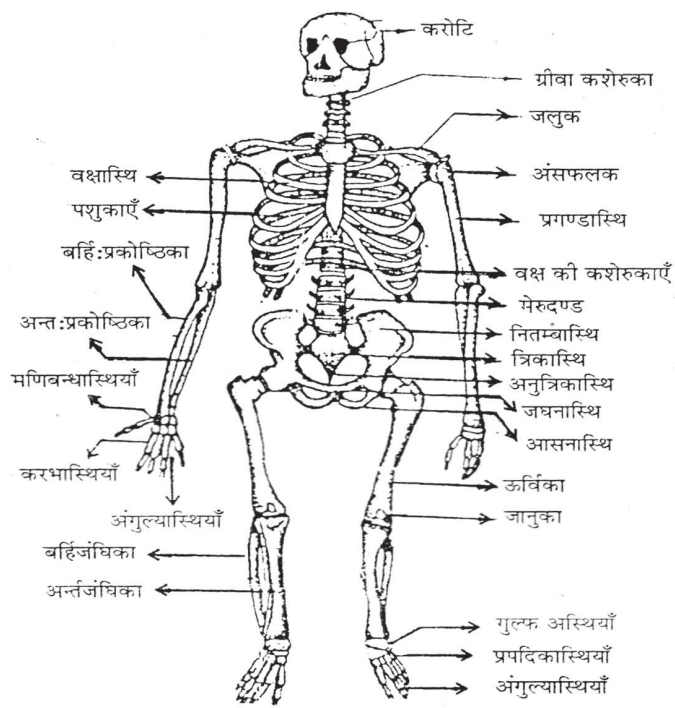
चित्र—मानव कंकाल
