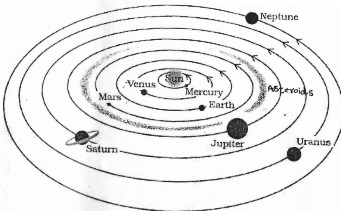
सौर परिवार
