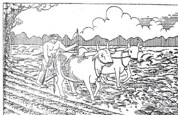
हल चलाना
