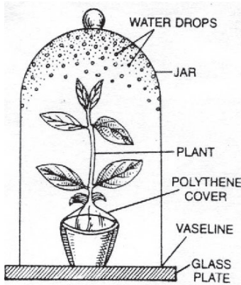
बेलजार विधि
