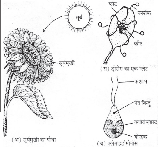
(ब) क्लेमाइडोमोर्नास
