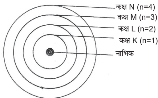
किसी परमाणु में ऊर्जा स्तर
