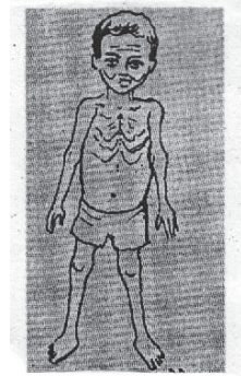
मेरेस्मस
