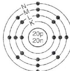
कैल्सियम-40
