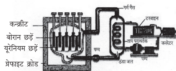
चित्र - परमाणु भट्टी
